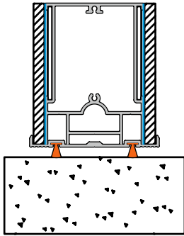
No Threshold Χωρίς Κατωκάσι Senza Soglia
