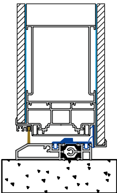
T4 Bottom Threshold Με κατωκάσι Con soglia
