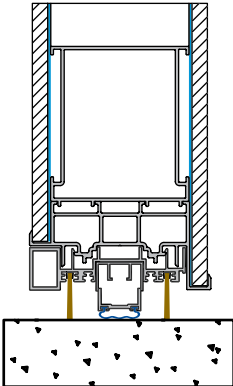
T5 Airstopper (No Threshold) Χωρίς κατωκάσι με αεροστόπ Senza soglia con parafreddo
