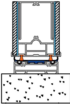
Bottom Threshold Με Κατωκάσι Con Soglia
